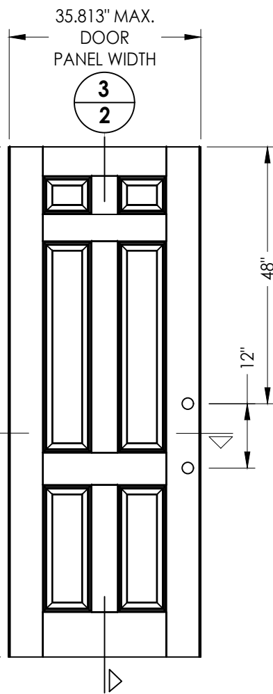
41 DOOR PANEL Hybrid Door
